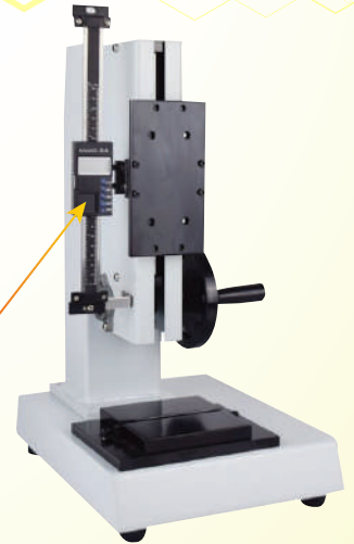
รุ่น ESC-500 พร้อมสเกลวัดระยะ (ESC-S)
